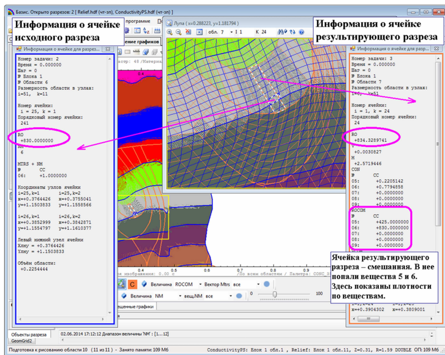
Рис. 12. Просмотр информации в ячейках разреза-источника и результирующего разреза, попадающих в заданную точку пространства разрезов (пунктиром выделены пересекающиеся ячейки)
