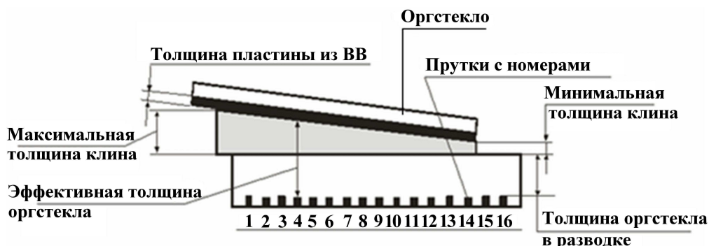
Рис. 6. Схема модели со встречным движением УВ и ДВ
