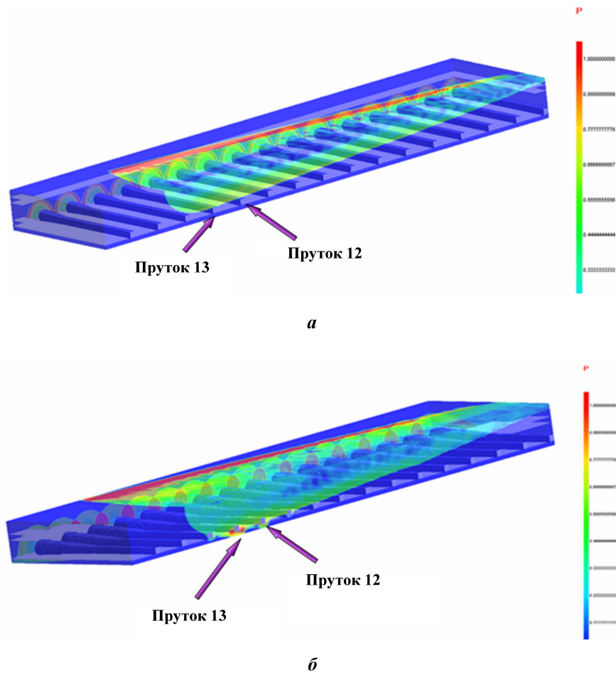
Рис. 11. Распределение давления в оргстекле: a – t = 5,5 мкс; б – t = 7 мкс
