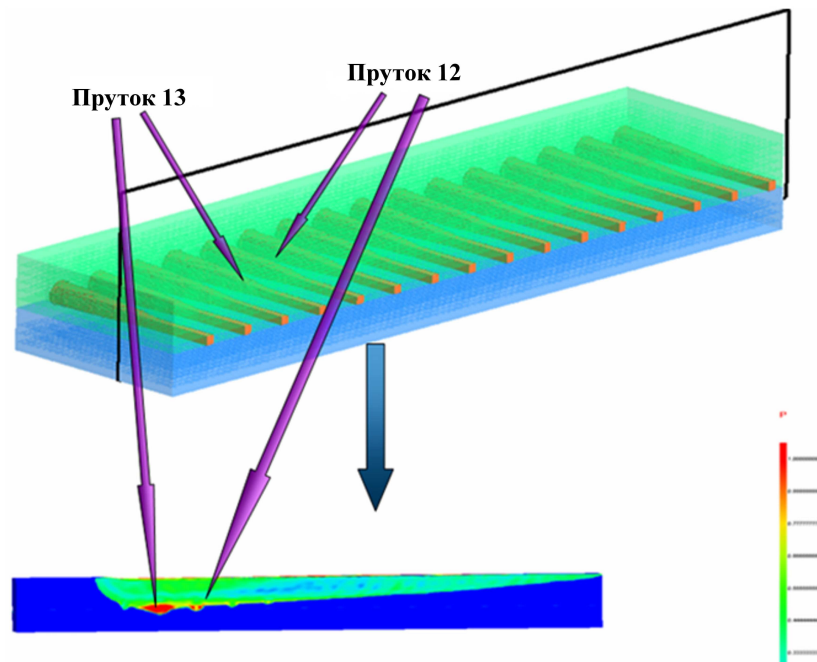
Рис. 12. Распределение давления в одном из сечений математической области задачи, t = 8 мкс
