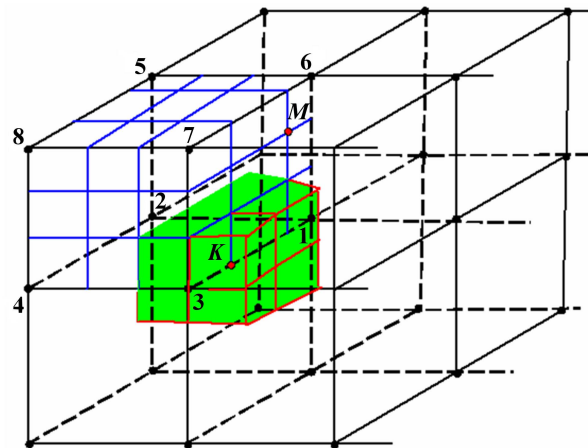
Рис. 5. Построение фиктивных адаптивных ячеек для аппроксимации уравнения движения в узле адаптивной сетки на границе структурированной и адаптивной сеток
