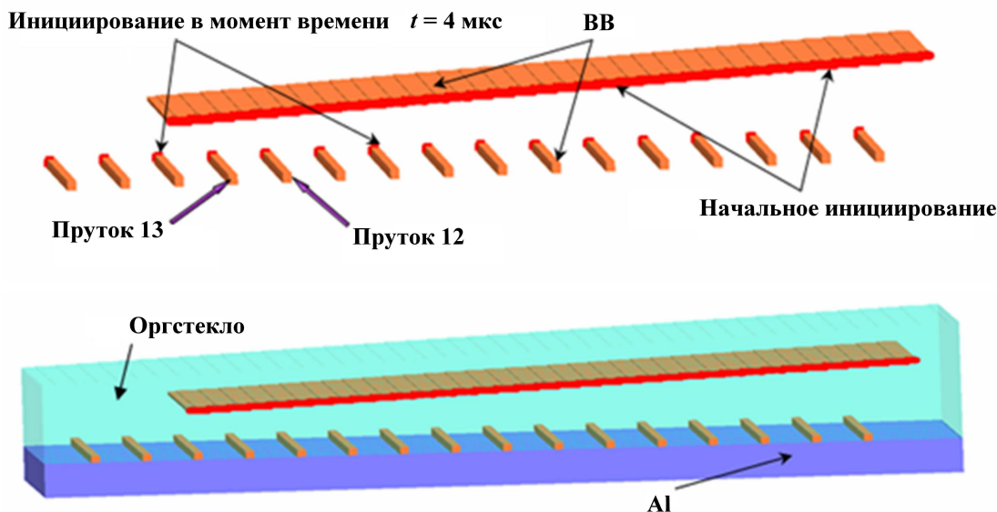
Рис. 8. Геометрия расчетов
