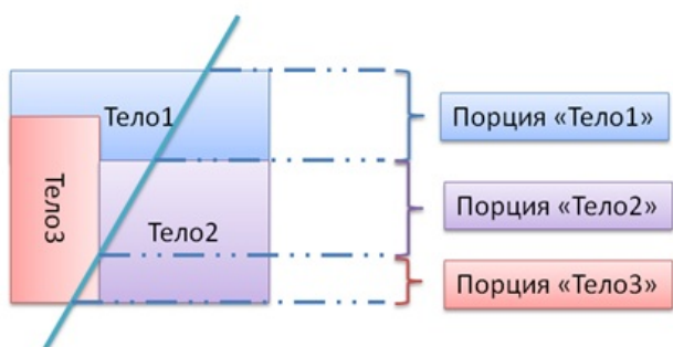
Рис. 2. Разбиение прямой линии на порции
