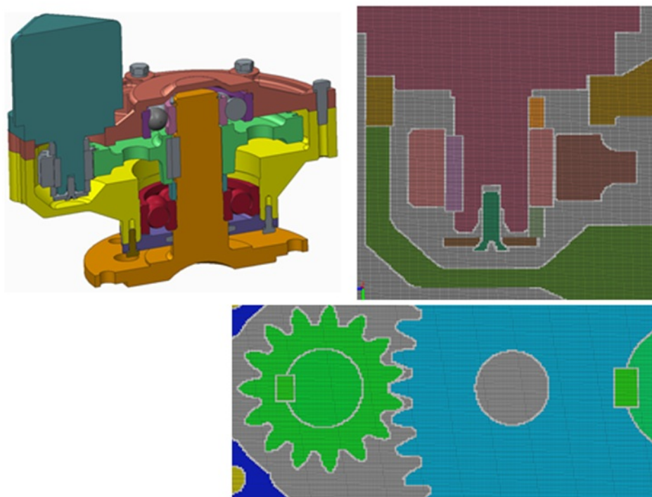
Рис. 3. Геометрическая модель и фрагменты прямоугольной структурированной сетки с рассчитанными объемными концентрациями
