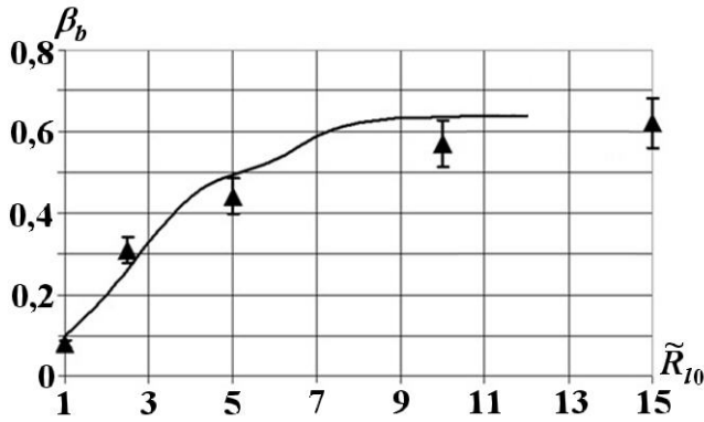
Рис. 11. Зависимости скорости роста амплитуды ЛВ от \tilde{R}_{10} на начальной стадии: — — расчет; \blacktriangle — эксперимент
