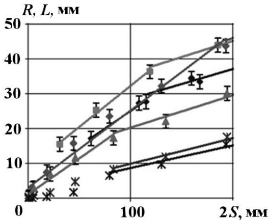
Рис. 12. Развитие амплитуды ЛВ и глубины проникания легкого вещества в тяжелое в ЗТП (эксперименты [15], фрагмент): \blacklozenge — R_{10} = 3 мм; \blacksquare — R_{10} = 6 мм; \circ — R_{10} = 6 мм; \blacktriangle — R_{10} = 2 мм; \ast — глубина проникания ЗТП (результаты двух экспериментов); \bar{I} — погрешность
