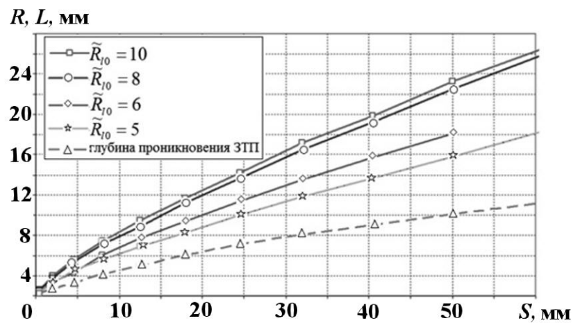
Рис. 10. Расчетные зависимости амплитуды ЛВ и глубины проникания легкого вещества в тяжелое в ЗПТ
