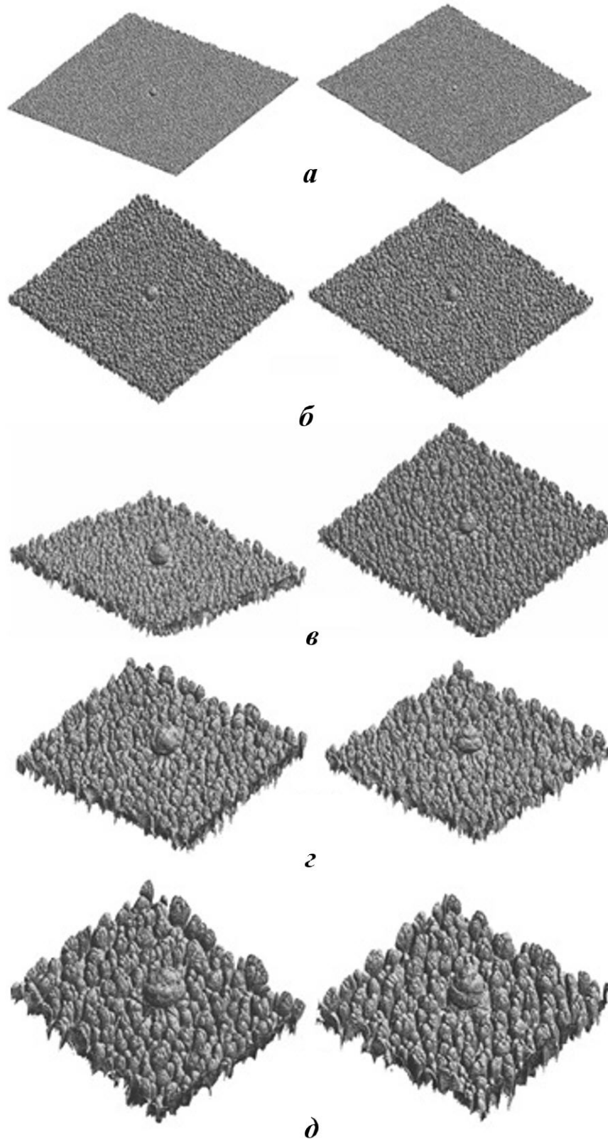
Рис. 6. Картины ЛВ и ЗТП на различные моменты времени при \tilde{R}_{l0} = 10 (слева) и \tilde{R}_{l0} = 8 (справа): a — S = 2 мм; б — S = 8 мм; в — S = 18 мм; г — S = 32 мм; д — S = 50 мм
