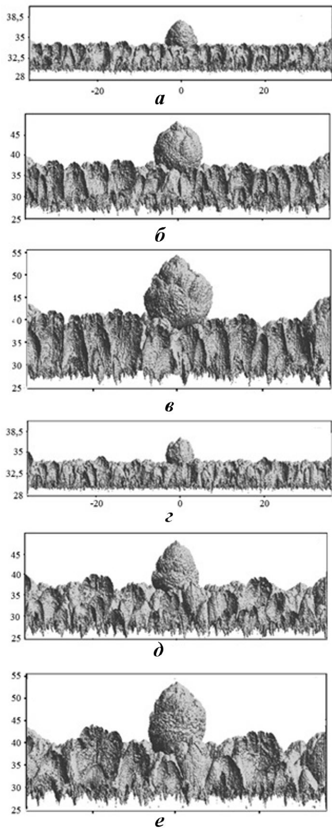
Рис. 8. Развитие ЛВ с \tilde{R}_{l0} = 10 (а-в) и \tilde{R}_{l0} = 8 (г-е): а — S = 18 мм; б — S = 40,5 мм; в — S = 60,5 мм; г — S = 18 мм; д — S = 40,5 мм; е — S = 60,5 мм
