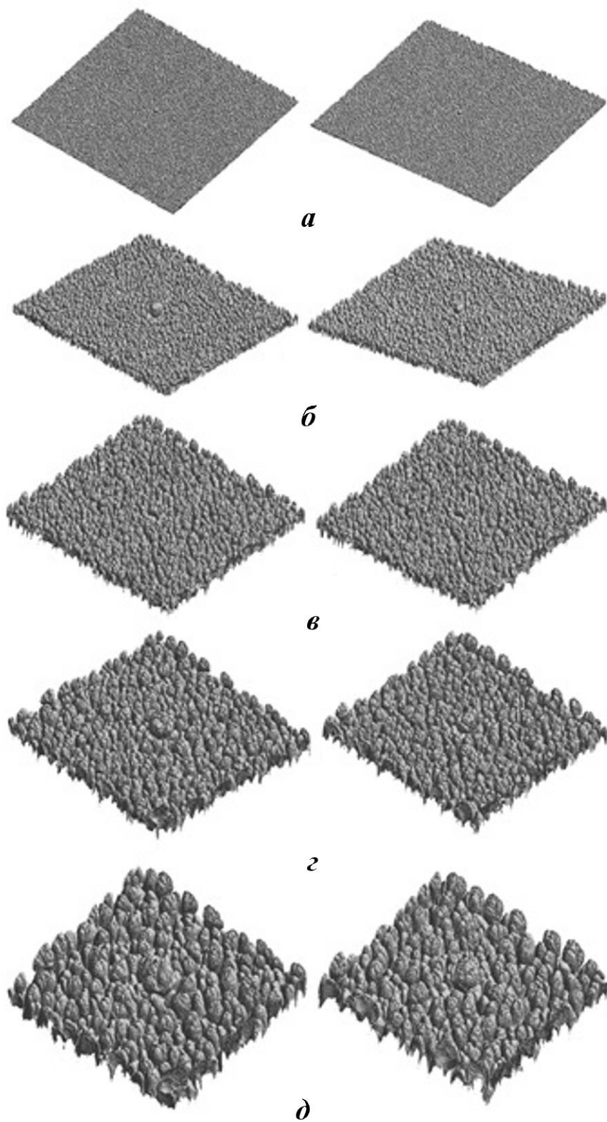
Рис. 7. Картины ЛВ и ЗТП на различные моменты времени при \tilde{R}_{l0} = 6 (слева) и \tilde{R}_{l0} = 5 (справа): а — S = 2 мм; б — S = 8 мм; в — S = 18 мм; г — S = 32 мм; д — S = 50 мм
