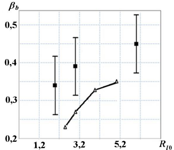
Рис. 13. Зависимости скорости роста амплитуды ЛВ от R_{10} на второй стадии процесса: \blacktriangle — расчет; \blacksquare — эксперимент; \bar{I} — погрешность
