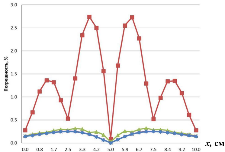
Рис. 13. Задача 1. Сходимость итерационного процесса на верхней границе области: —■— — итерационная коррекция, 1 итерация; —▲— — итерационная коррекция, 2 итерации; —×— — итерационная коррекция, 3 итерации; —◆— — аналитическая коррекция
