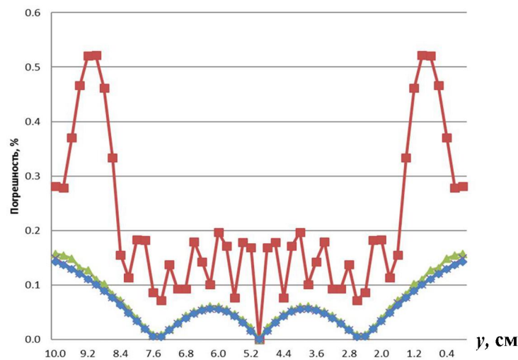
Рис. 14. Задача 1. Сходимость итерационного процесса на правой границе области: —■— — итерационная коррекция, 1 итерация; —▲— — итерационная коррекция, 2 итерации; —×— — итерационная коррекция, 3 итерации; —◆— — аналитическая коррекция
