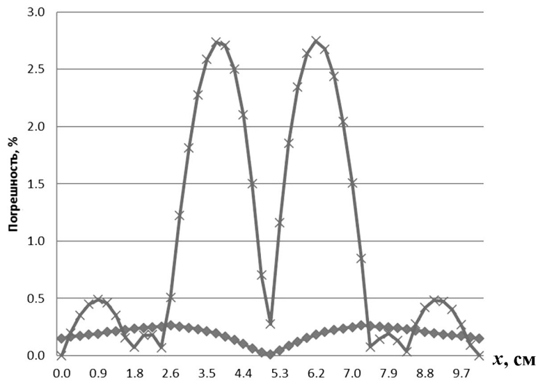
Рис. 11. Задача 1. Сравнение погрешностей для базового алгоритма с окрестностью 4 (—x—) и алгоритма с итерационной коррекцией (—♦—) на верхней границе области
