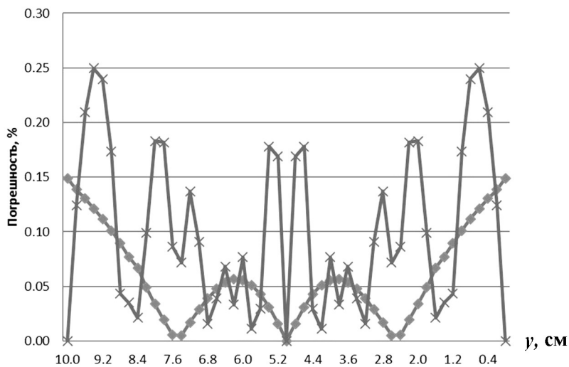
Рис. 12. Задача 1. Сравнение погрешностей для базового алгоритма с окрестностью 4 (—x—) и алгоритма с итерационной коррекцией (—♦—) на правой границе области
