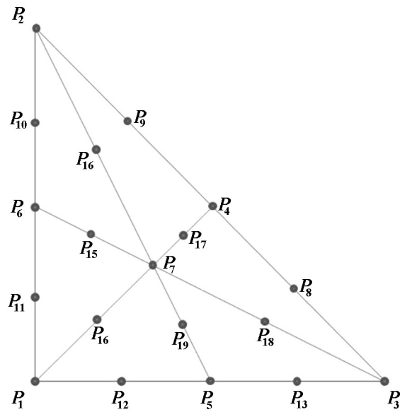
Рис. 6. Схема разбиения треугольника
