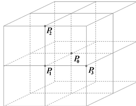
Рис. 5. Фрагмент трехмерной кубической счетной сетки
