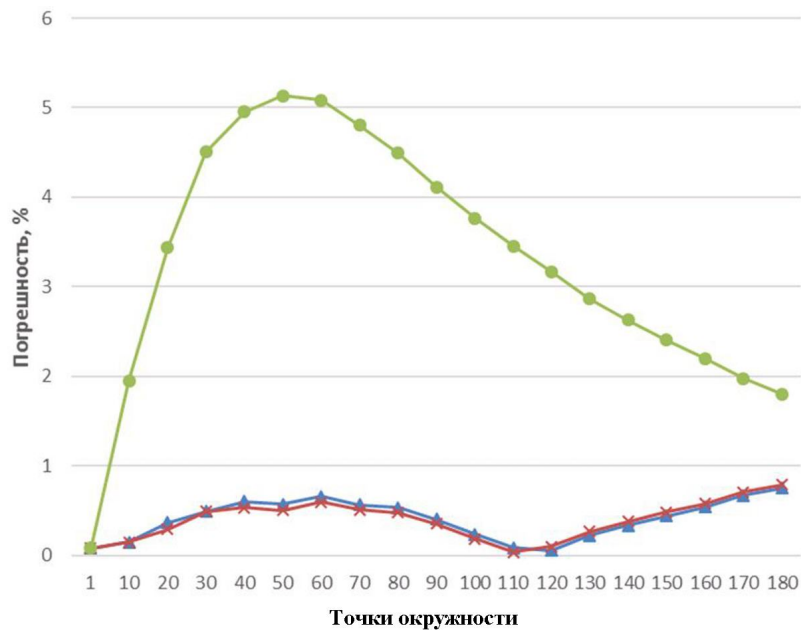
Рис. 17. Задача 3. Погрешность времен детонации на внутренней границе ВВ: \text{—}\blacktriangle\text{—} — итерационная коррекция; \text{—}\times\text{—} — аналитическая коррекция; \text{—}\bullet\text{—} — базовый алгоритм, окрестность 4
