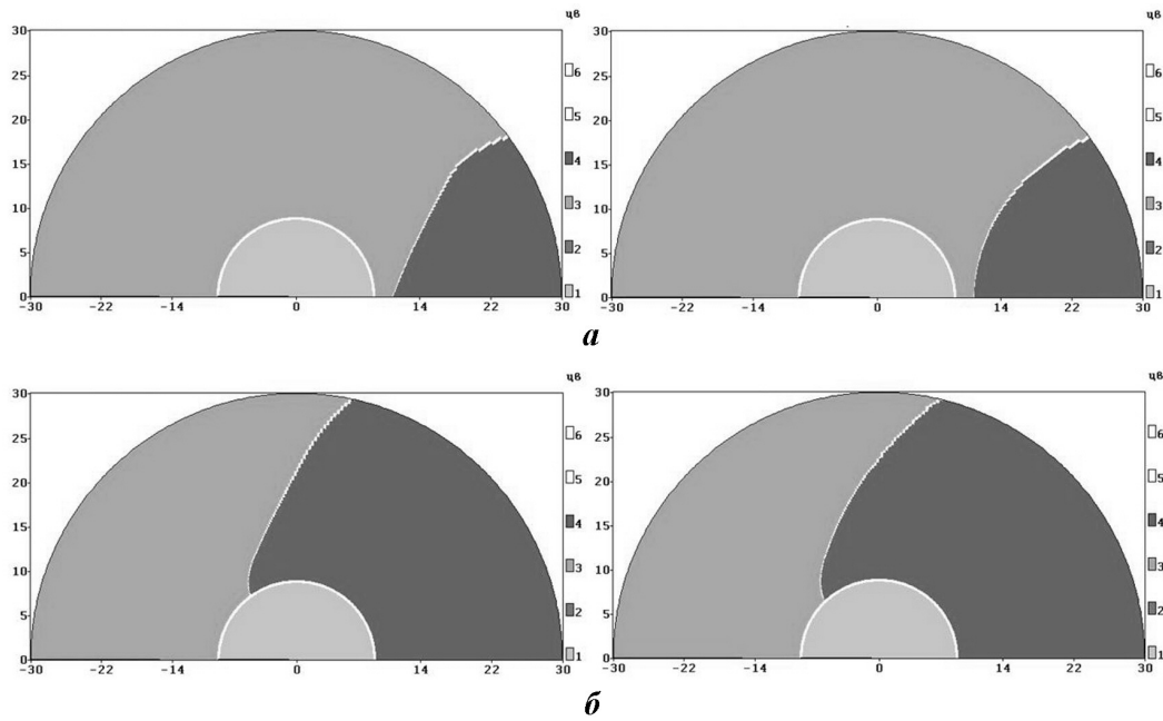
Рис. 16. Задача 3. Фронт ДВ для базового алгоритма с окрестностью 4 (слева) и алгоритма с итерационной коррекцией (справа): a - t = 25 \text{ мкс} ; б - t = 50 \text{ мкс}
