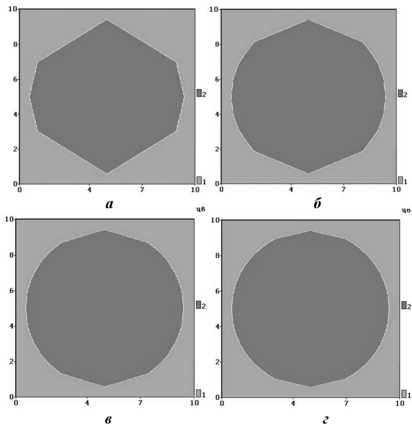
Рис. 7. Задача 1. Фронт сферической ДВ на момент времени t = 5 мкс для базового пошагового алгоритма с различными размерами окрестности влияния: a — окрестность 1; б — окрестность 2; в — окрестность 3; г — окрестность 4
