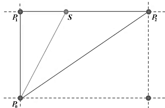
Рис. 3. Фрагмент двумерной счетной сетки
