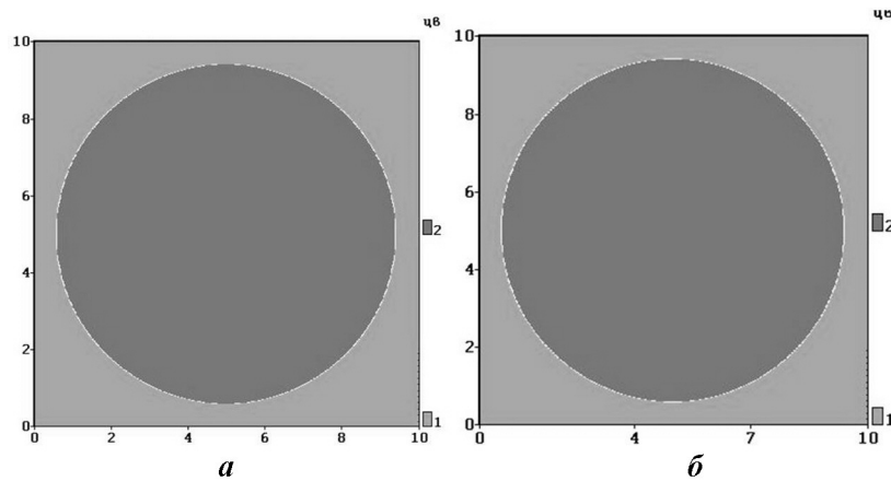
Рис. 10. Задача 1. Фронт сферической ДВ на момент времени t = 5 мкс для окрестности 1 с аналитической (а) и итерационной (б) коррекцией времен детонации
