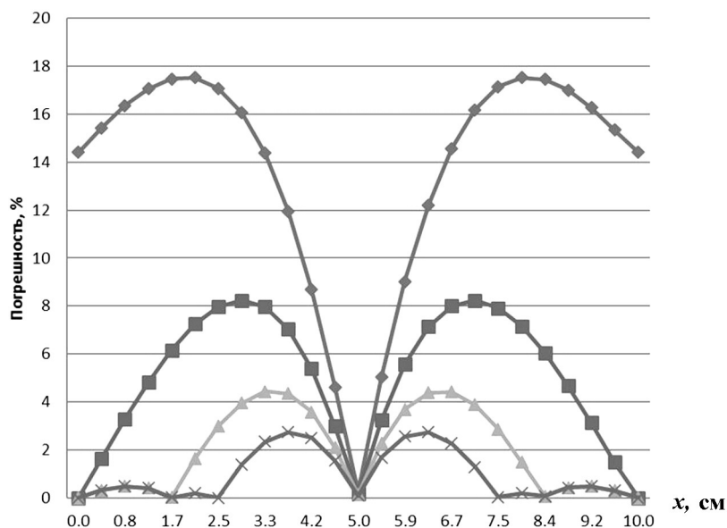
Рис. 8. Задача 1. Сравнение погрешностей на верхней границе области для базового алгоритма с различными размерами окрестности влияния: —♦— — окрестность 1; —■— — окрестность 2; —▲— — окрестность 3; —×— — окрестность 4
