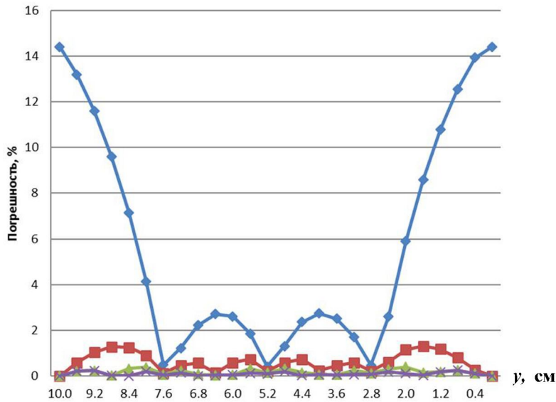
Рис. 9. Задача 1. Сравнение погрешностей на правой границе области для базового алгоритма с различными размерами окрестности влияния: —♦— окрестность 1; —■— окрестность 2; —▲— окрестность 3; —×— окрестность 4
