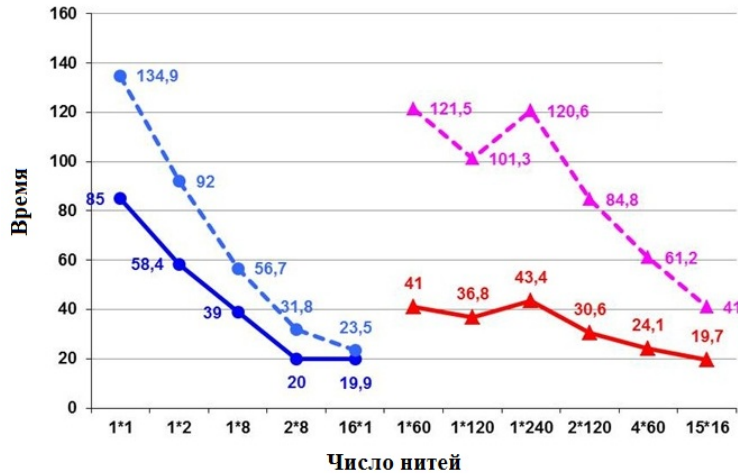
Рис. 1. Время решения ста СЛАУ задачи AV13: \blacktriangle -, \text{---}\blacktriangle --- — сопроцессор; \bullet -, \text{---}\bullet --- — ЦП
