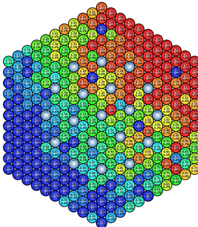
Рис. 11. Отклонения результатов расчета по программе TDMCC от результатов по MCNP для ТВС P40E9 № 2
