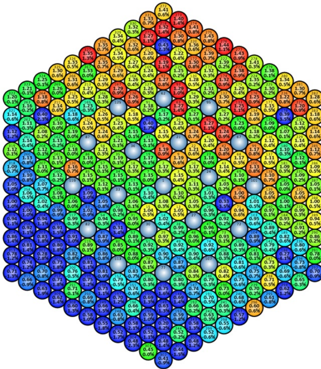
Рис. 12. Отклонения результатов расчета по программе TDMSS от результатов по MCNP для ТВС РЗБЕ9 № 3
