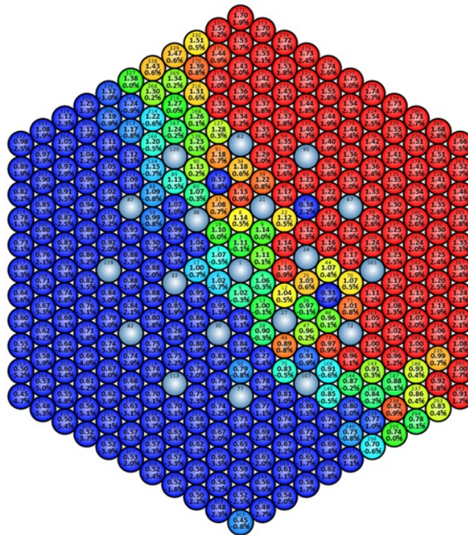
Рис. 10. Отклонения результатов расчета по программе TDMCC от результатов по MCNP для ТВС А40Е6 № 1
