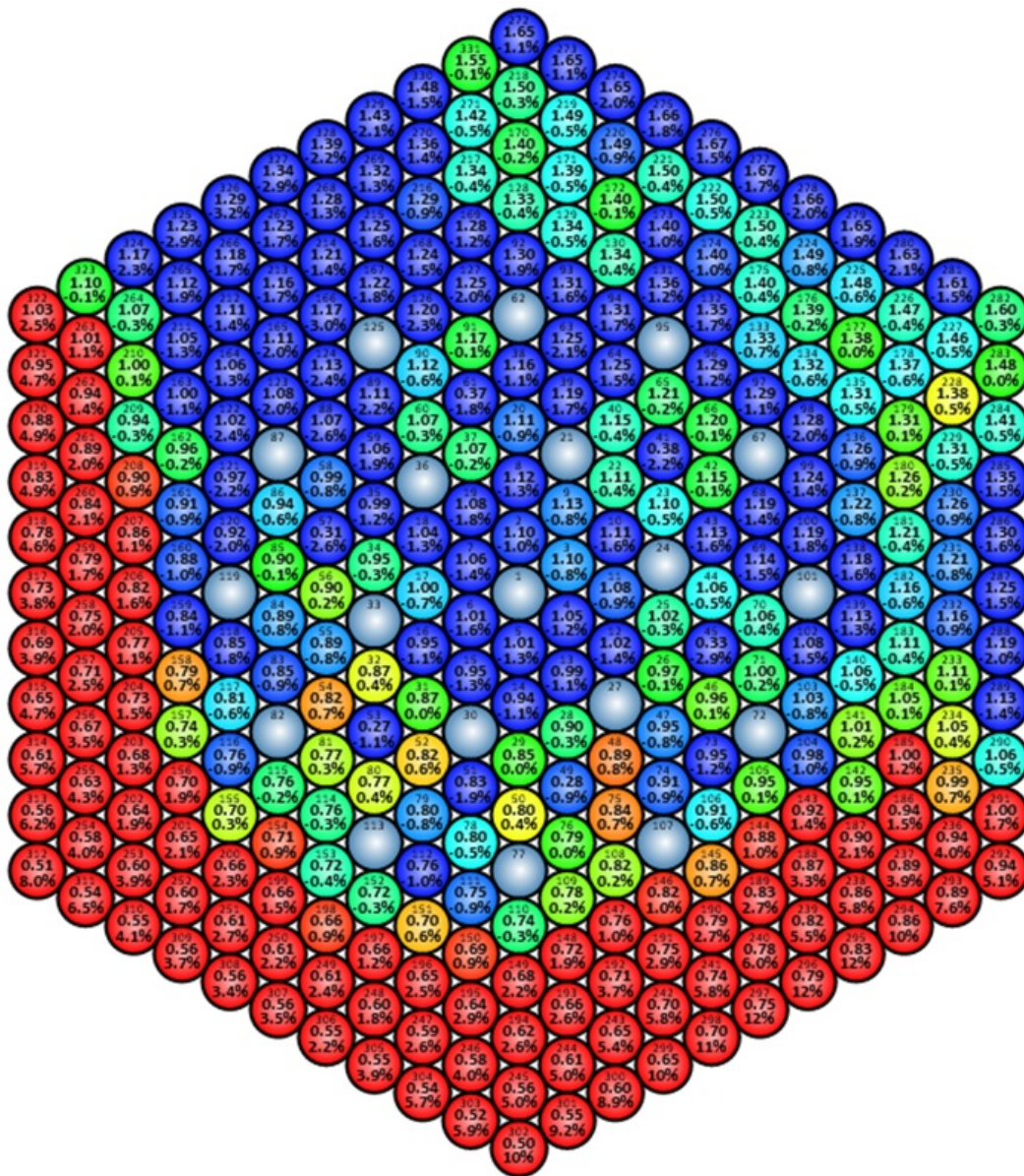
Рис. 16. Расчет мелкосеточным методом с шестью группами нейтронов. Относительное отклонение результатов расчета по программе TDMCC от результатов по САФИР_95&RC_VVЭР в твэлах ТВС № 1 (тип А40Е6)
