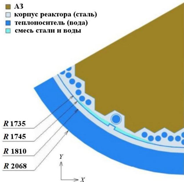
Рис. 1. Горизонтальное сечение 1/6 корпуса реактора, окружающего АЗ
