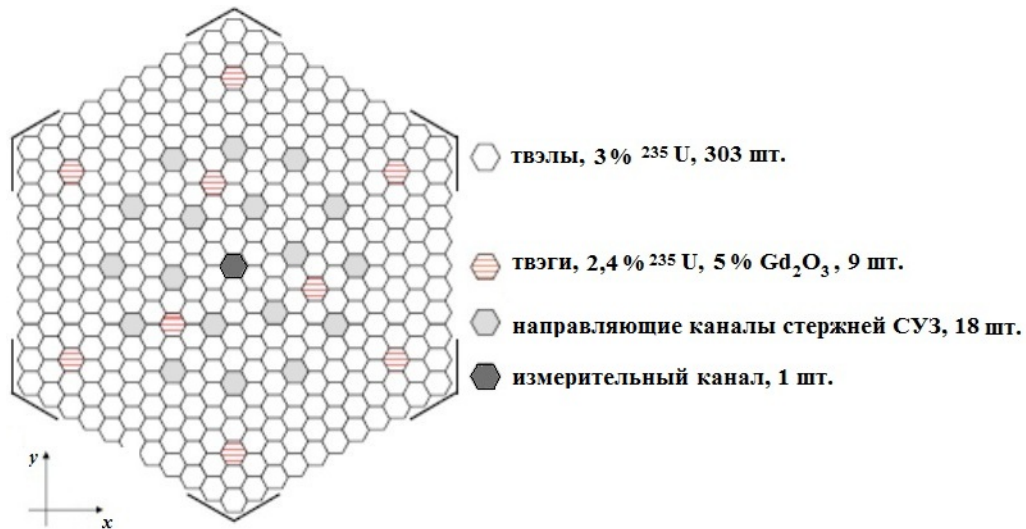
Рис. 4. ТВС типа А40Е6
