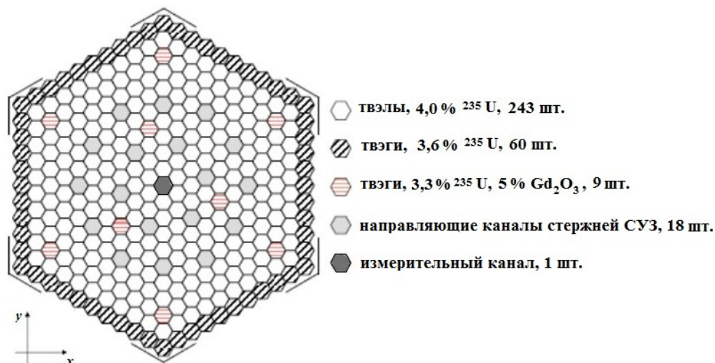
Рис. 7. ТВС типа P40E9
