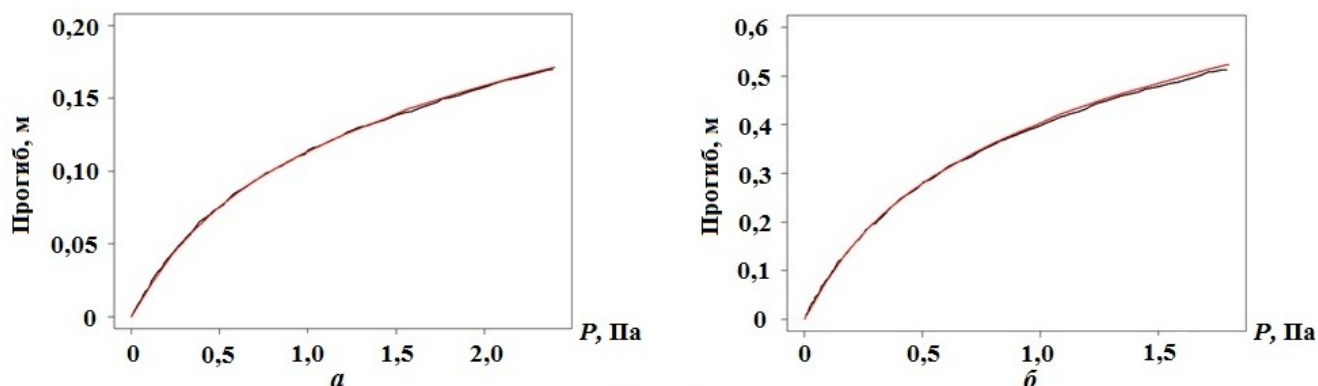
Рис. 2. Зависимости прогиба в центре пластины от давления для композитов А (а) и Б (б): — — эталон; — — ПП "Логос"
