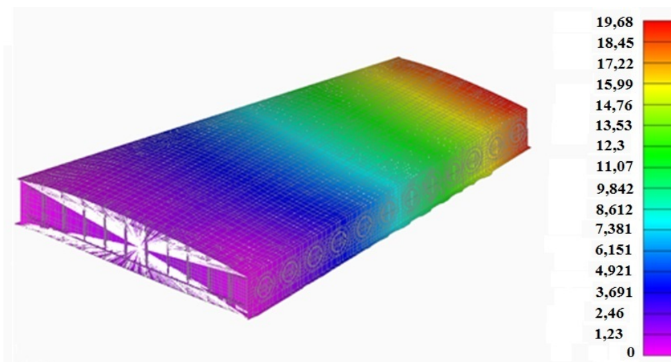
Рис. 5. Поле результирующих перемещений в задаче расчета НДС панели по КПО "Nastran"
