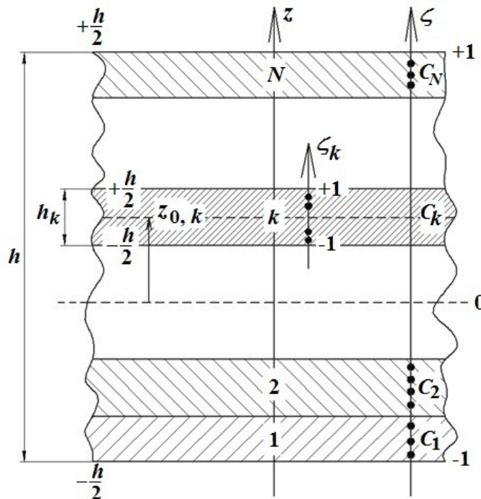
Рис. 1. Модель многослойного КМ в модуле "Логос Прочность"
