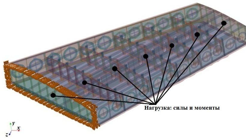
Рис. 3. Постановка задачи расчета НДС панели
