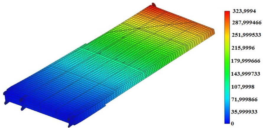
Рис. 7. Поле результирующих перемещений в задаче расчета НДС панели из КМ по ПП "Логос"
