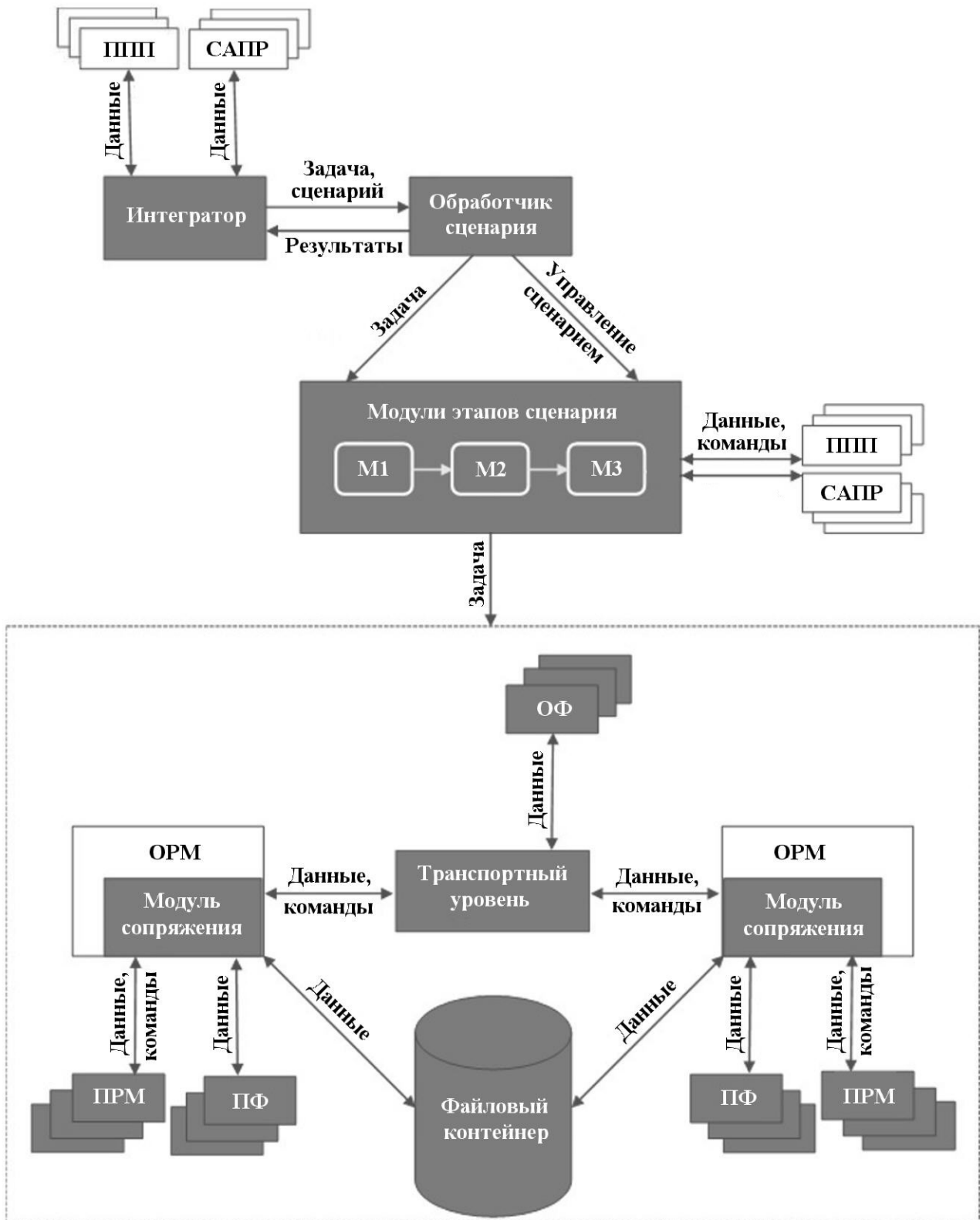
Рис. 1. Схема взаимодействия компонентов ПМ "Логос Платформа" 2
