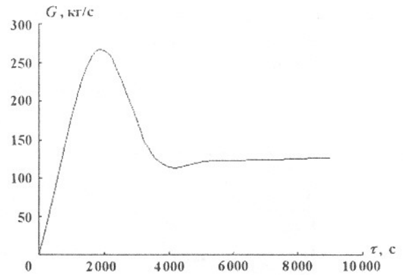
Рис. 3. Изменение расхода натрия через реактор во времени в случае расплавления 36 ТВС
