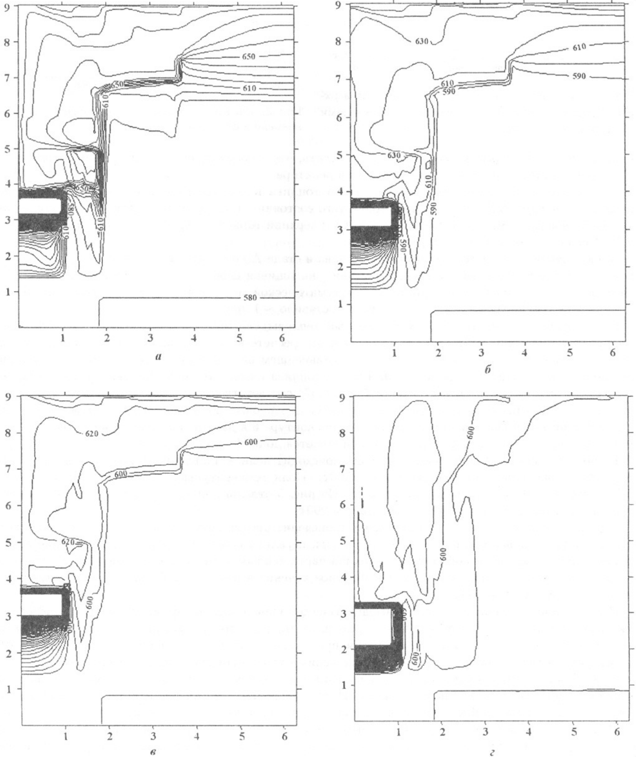
Рис. 4. Поле температуры: а - \tau = 3600 с; б - \tau = 7200 с; в - \tau = 10800 с; з - \tau = 54100 с
