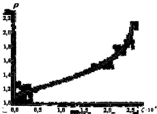
Рис. 8. Распределение плотности по координате (в безразмерных переменных)
