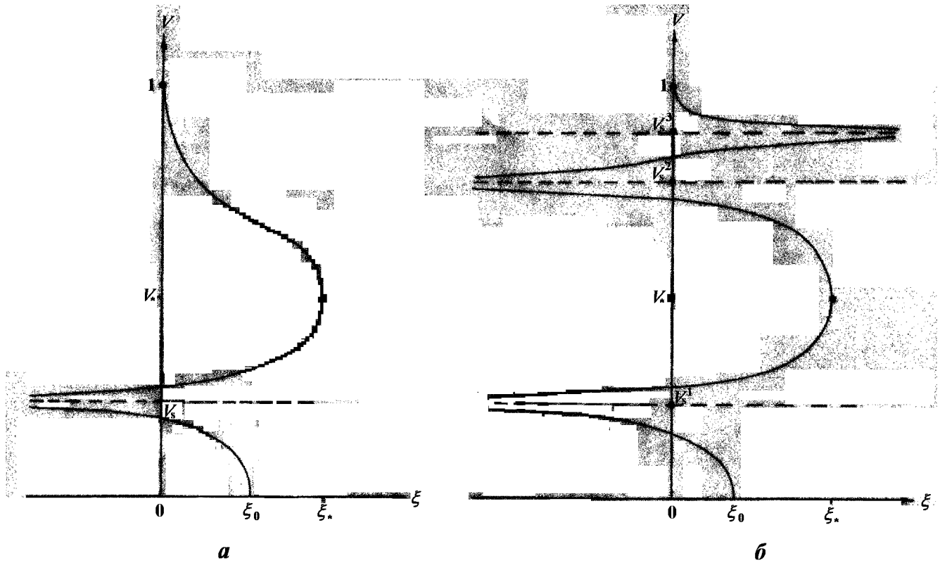
Рис. 4. Структура решения при положительном тепловом потоке в критической точке: a — вариант с одной точкой покоя; b — вариант с тремя точками покоя
