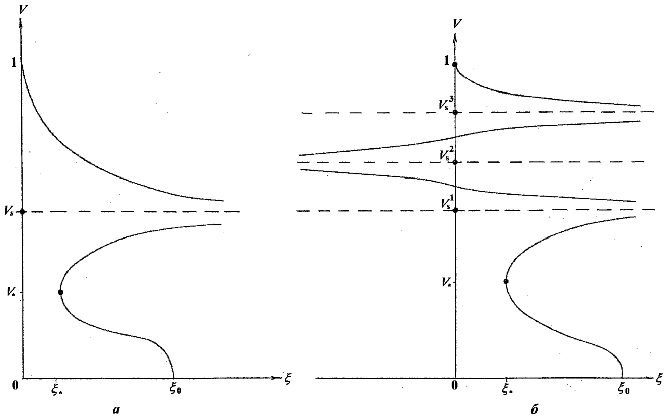
Рис. 5. Структура решения при отрицательном тепловом потоке в критической точке: a — вариант с одной точкой покоя; б — вариант с тремя точками покоя
