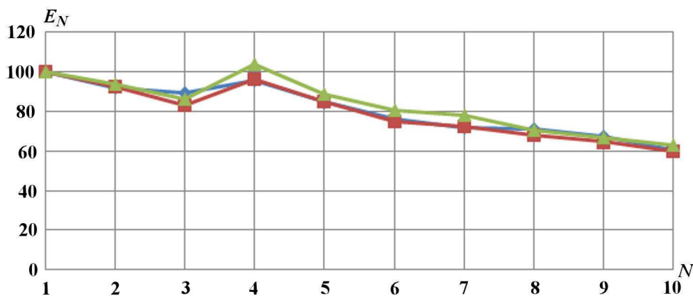
Рис. 2. Зависимости эффективности распараллеливания от количества потоков для сеток разного размера:
