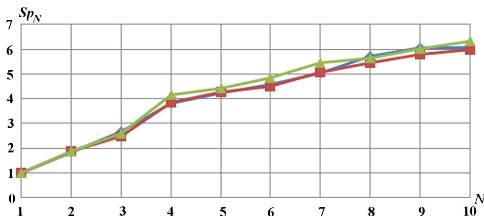
Рис. 3. Зависимости коэффициента ускорения от количества потоков для сеток разного размера:
