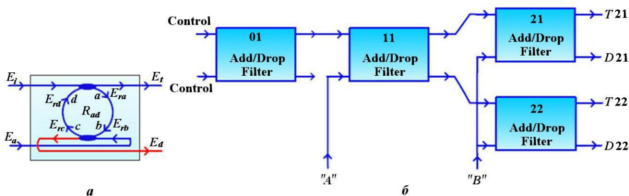
Рис. 5. Схемы МКР (а) и ОЛЭ NAND (б) из [31]
