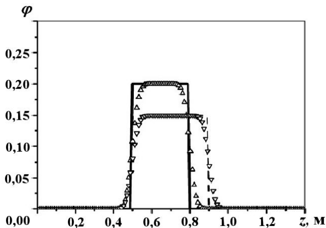
Рис. 4. Перенос частиц стали и топлива: — — аналитическое решение для стали; \Delta — расчет с помощью кода ЕВКЛИД/V2 для частиц стали; — — — аналитическое решение для топлива; \nabla — расчет с помощью кода ЕВКЛИД/V2 для частиц топлива
