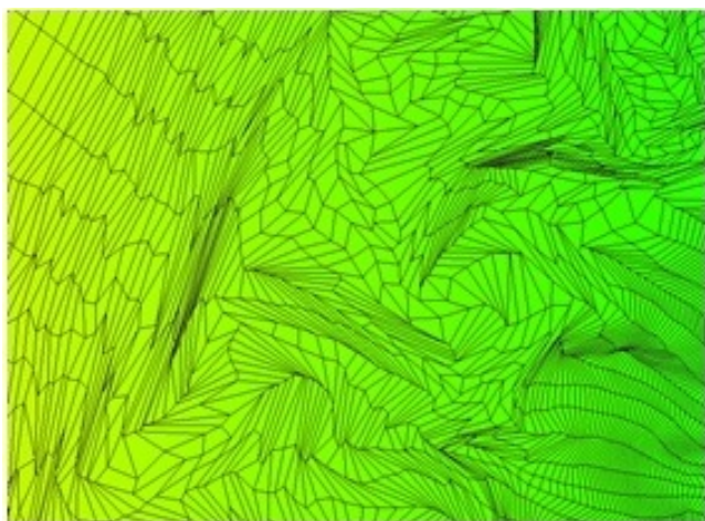
Рис. 1. Искаженная сетка
