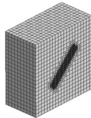
Рис. 6. Результат генерации дробно-адаптивного шаблона
