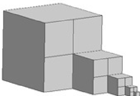
Рис. 7. Формирование ячеек
