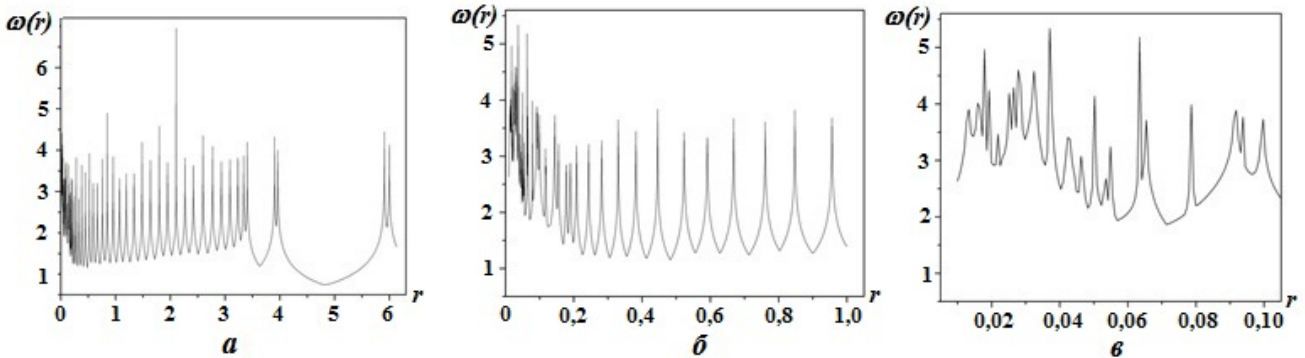
Рис. 2. Спектральные портреты матрицы A_{100} для разных диапазонов изменения радиуса r : a — 0 < r < 6 ; b — 0 < r < 1 ; c — 0 < r < 0,1
